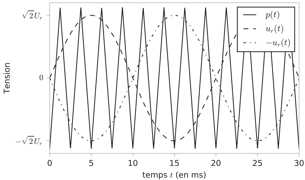
FIGURE 5 – Représentation des fonctions de commande p , u_r et -u_r en fonction du temps pour l'onduleur à commande décalée. Ce graphique est donné à titre indicatif afin d'aider le candidat si besoin.
