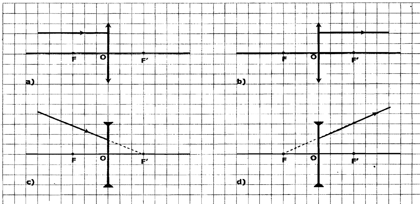
Figure 1 : Marche de rayons lumineux à travers des lentilles minces
